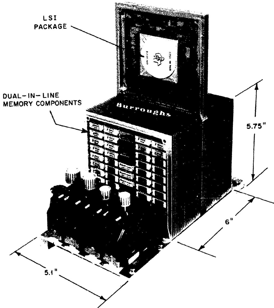
Figure 30. Interpreter Module Packaging
